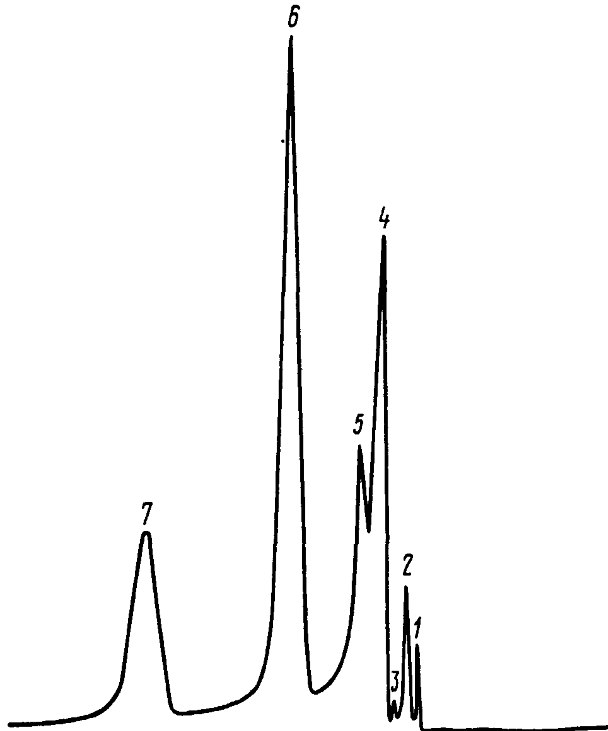
Типовая хроматограмма технической муравьиной кислоты
